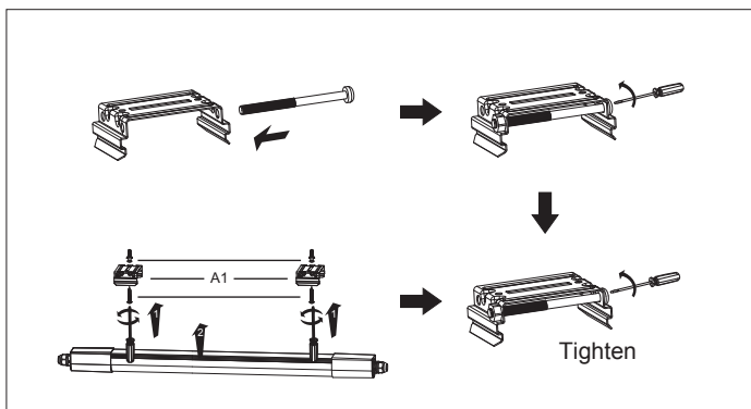
Tarvikkeet varkaudenestoon (saatavana erikseen) LA10195
