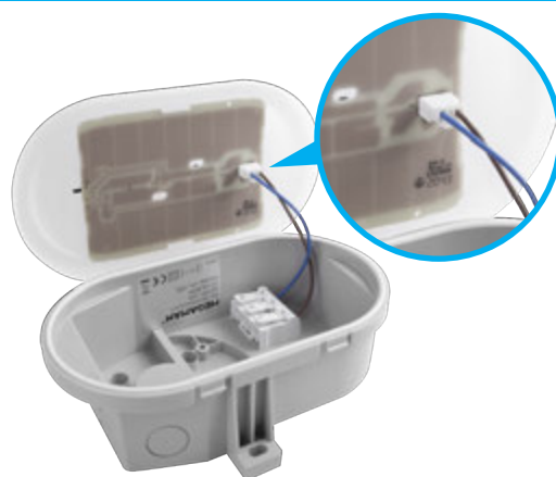
Helppo ja nopea asennus pikaliittimellä
